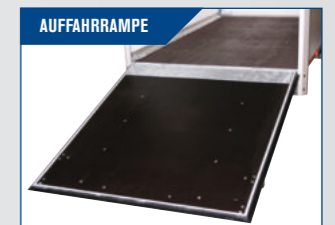
AUFFAHRAMPE Extra verstärkt. Kann anstatt Doppeltüren hinten gegen Aufpreis gewählt werden.
